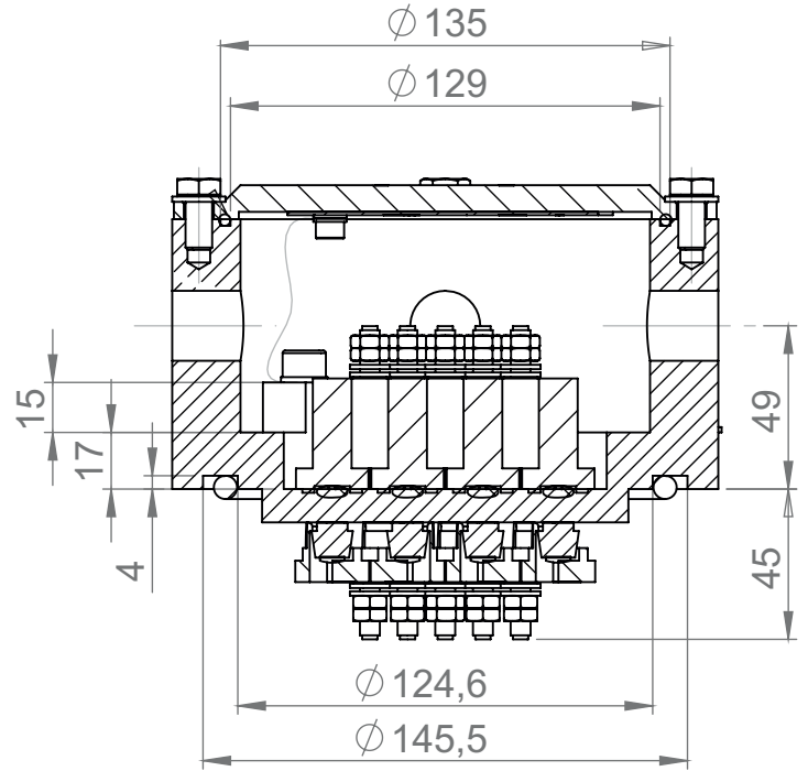
C-C (1 : 2.5)
